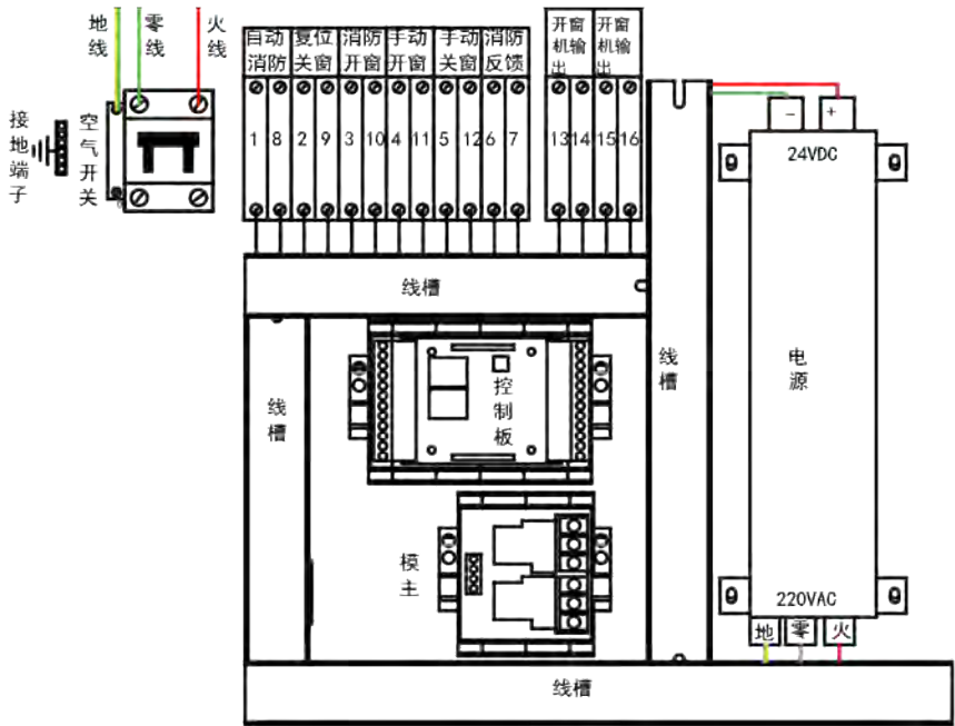
接线图
